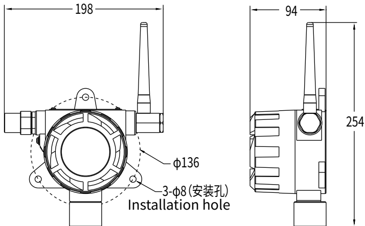
尺寸图 Physical Dimensions
