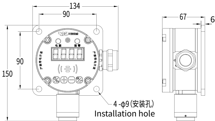
尺寸图 Physical Dimensions
