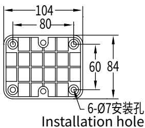
尺寸图 Physical Dimensions
