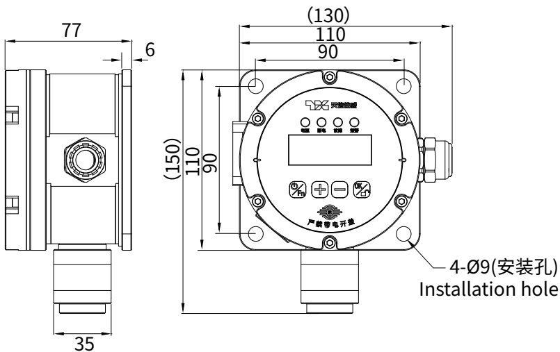
尺寸图 Physical Dimensions
