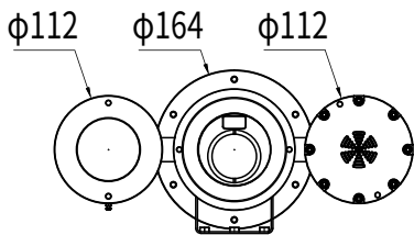
尺寸图 Physical Dimensions
