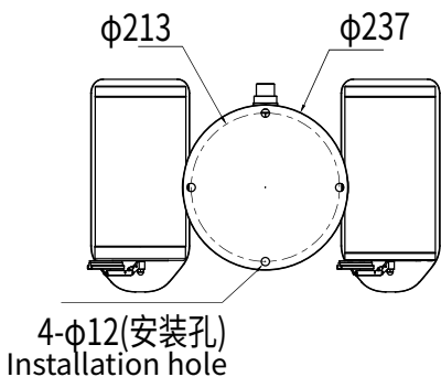
尺寸图 Physical Dimensions
